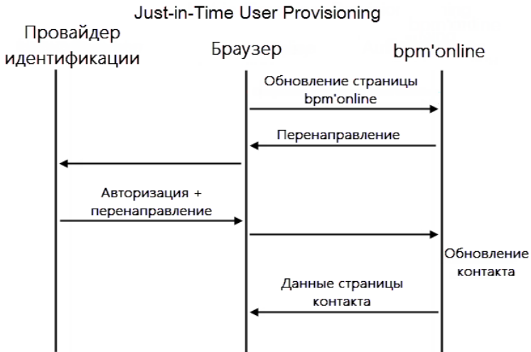
Рис. 350 — Схема обновления данных при использовании Just-in-Time User Provisioning
